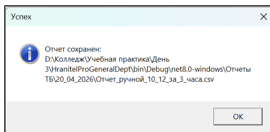
Рисунок 7 – Сохранение отчета
